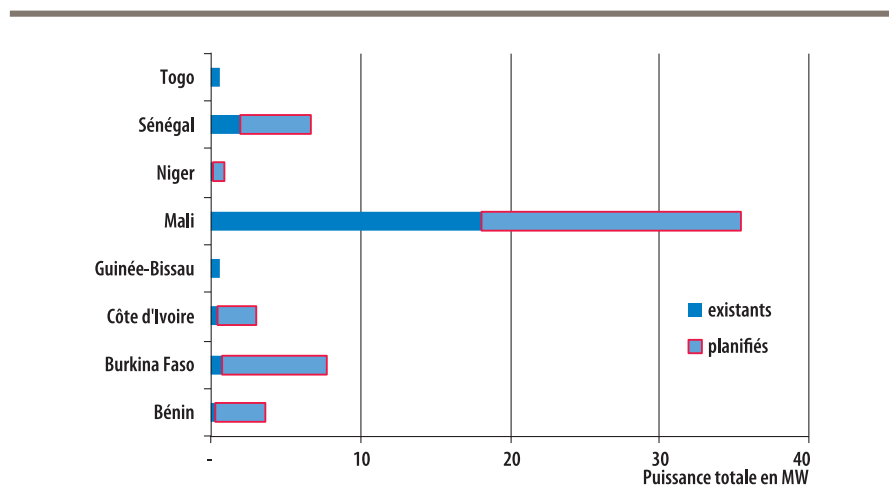
Figure 3. puissance totale des mini-réseaux existants et planifiés dans les pays membres de l'UEMOA (Source : ECREEE)
