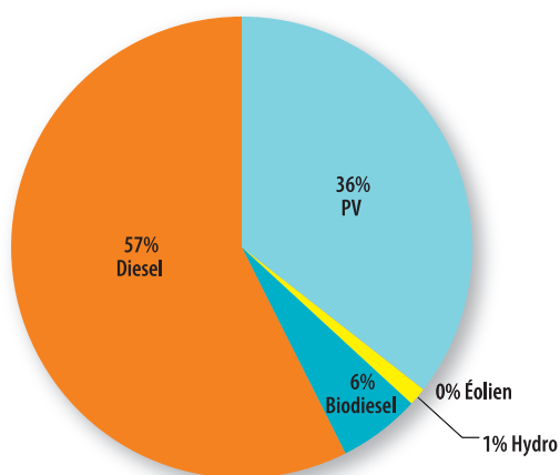
Figure 5. sources d'énergie des mini-réseaux (Source : ECREEE)
