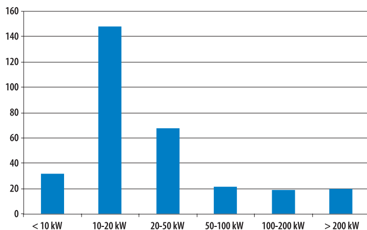
Figure 4. distribution des mini-réseaux recensés par catégorie de puissance (Source : ECREEE)
